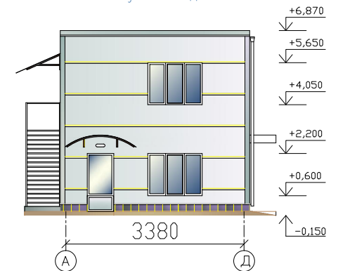
Фасад в осях А-Д
