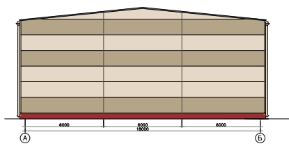
Фасад А-Б
